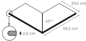
CANTO EXTERIOR BOLEADO SS 2 PEÇAS _ PIECES 29,4x59,2x2 cm P237 / peça_pieza
