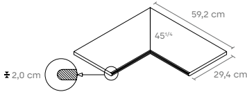
CANTO INTERIOR BOLEADO SS 2 PEÇAS _ PIECES 29,4x59,2x2 cm P237 / peça_pieza
