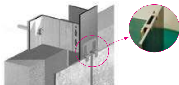
FACHADA COM GRAMPO À VISTA FACADES USING VISIBLE FASTENERS FAÇADE AGRAFÉE AVEC AGRAFE APPARENTE FACHADA CON GRAPA A LA VISTA
